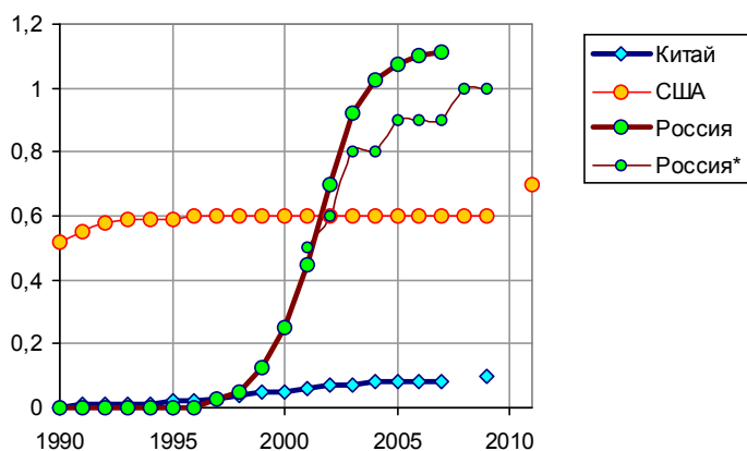
Доля ВИЧ-инфицированных среди населения
