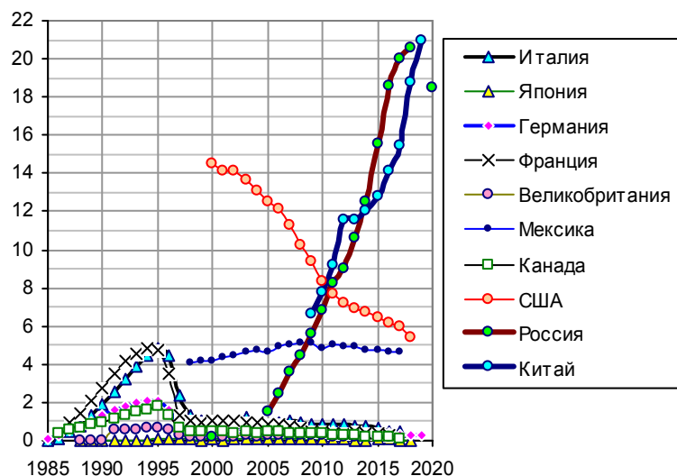
Количество умерших от ВИЧ - СПИД в некоторых странах, тысяч человек. Источник: OECD.Stat; CDC, NVSR; [I.24]; NBS.
