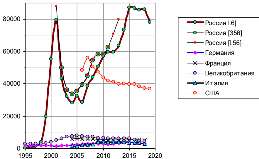
Количество граждан, инфицированных ВИЧ за год в РФ, США и в развитых странах Европы. Источники: [I.6, I.31, I.56, S.118]; European health for all databases (HFA-DB), WHO/Europe; CDC, HIV in United States.
