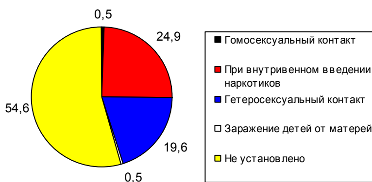
Распределение ВИЧ-инфицированных в России по основным факторам риска заражения в 2014 г., %. Источник: [1.56].
