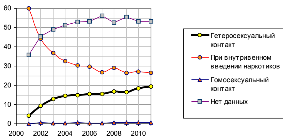
Распределение ВИЧ-инфицированных в России по основным факторам риска заражения, %. Источники: [1.56, 356].
