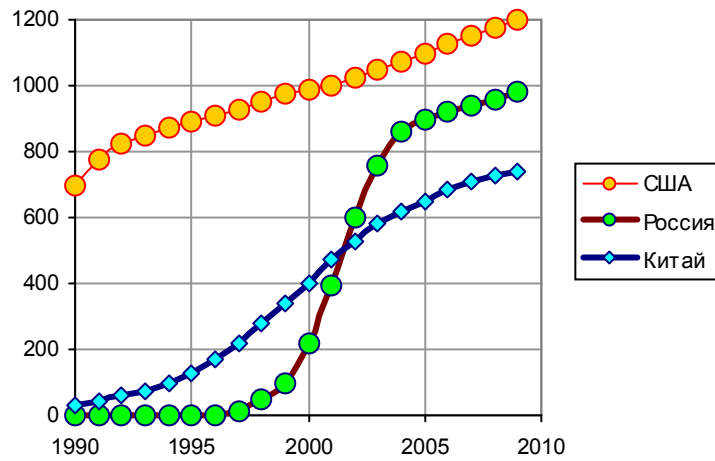
Оценка количества ВИЧ-инфицированных граждан, тысяч. Источник: WHO, UNAIDS.
