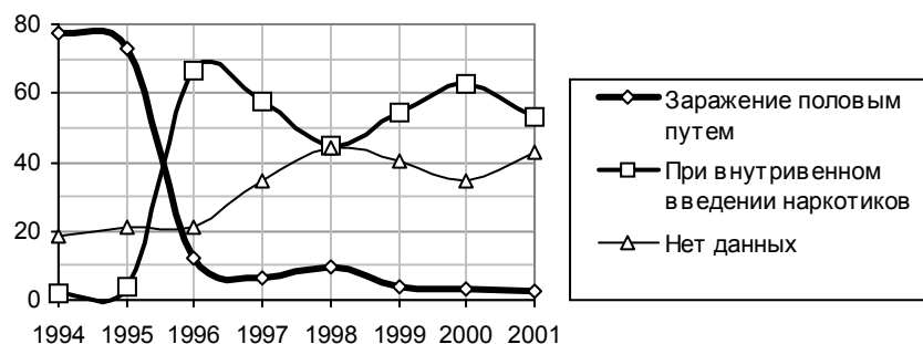
Распределение ВИЧ-инфицированных в России по основным факторам риска заражения, %. Источник: [144].
