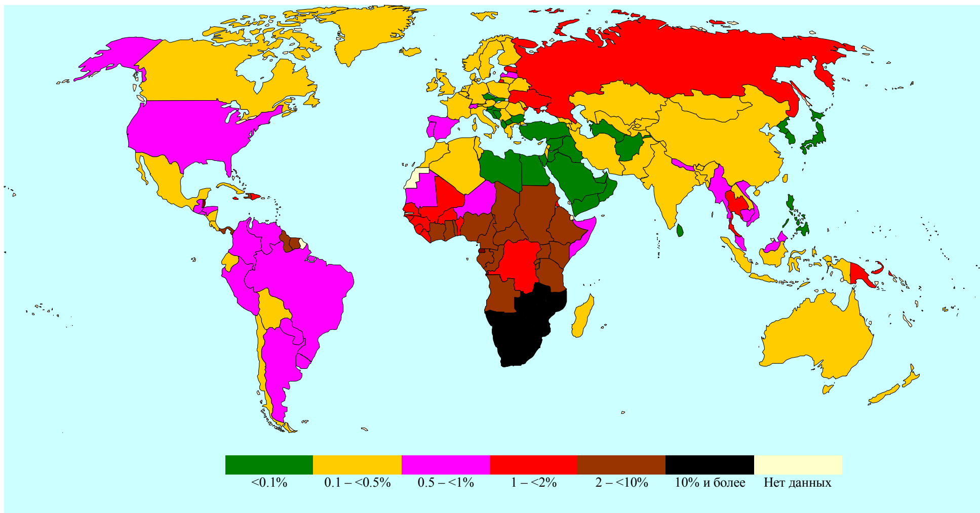
Оценка ВОЗ распространенности ВИЧ среди взрослого населения (15 – 49 лет) в 2007 году. Источники: построено по данным WHO, HIV and AIDS Estimates and Data, 2007 and 2001; CIA-The World Factbook.
