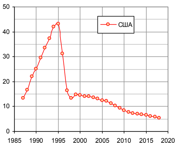
Количество умерших от ВИЧ – СПИД в США, тысяч человек. Источники: OECD.Stat; CDC, NVSR.
