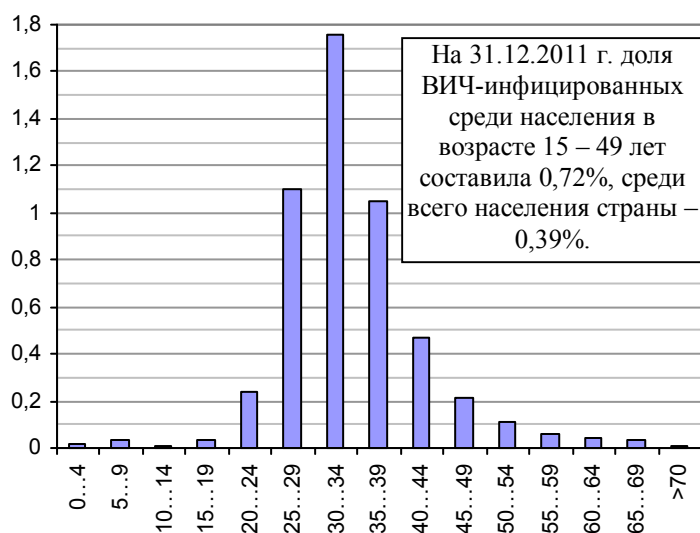
Пораженность населения РФ ВИЧ-инфекцией в различных возрастных группах на 21.12.2011, проценты. Источник: Федеральный центр СПИД, [356].
