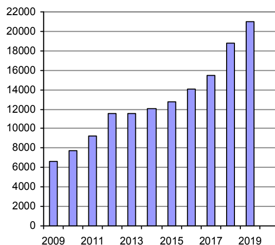
Количество умерших от СПИД в Китае, человек. Источник: China Statistical Yearbook.
