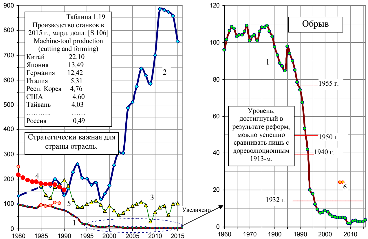
Рис. 1.156, а. Производство металлорежущих станков в России (1), Китае (для Китая не учитываются сверлильные, шлифовальные и полировальные станки, линия 2), Японии (metal cutting machine tools, линия 3), СССР (4) и в США (metal-cutting machines, линия 5; заказы и экспорт, линия 6) тыс. штук. Источники: National Bureau of Statistics of China; Statistics Bureau, Japan: Historical Statistics of Japan; Japan Statistical Yearbook; [I.3, I.4, I.6, I.57, S.89]; U.S. Census Bureau, The 2011 Statistical Abstract.
