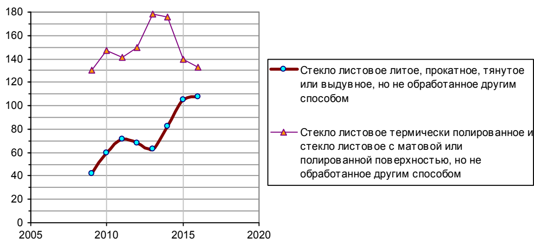
Рис. 1.187, а. Производство листового стекла в России, млн. м 2 . Источник: [1.6].
