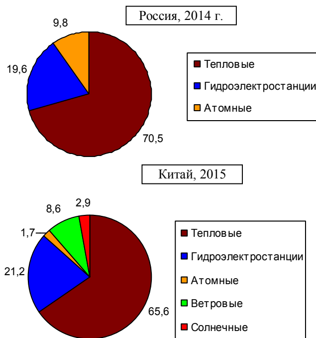
Рис. 1.124, б. Мощность электростанций РФ и Китая по типам, в процентах от общей мощности электростанций. Источники: [1.6]; National Bureau of Statistics of China.
