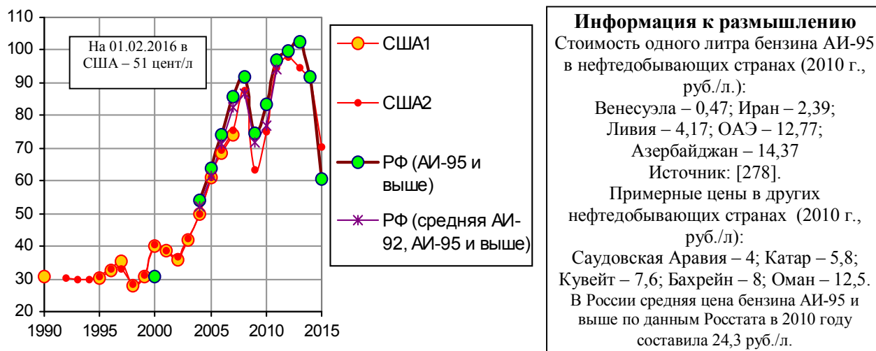
Рис. 4.5, а. Цена за 1 л бензина (unleaded regular) для конечного потребителя в США (линия США1), средняя розничная цена бензина всех марок в США (Gasoline All Grades Retail Price Including Taxes, U.S. Average, линия США2) и средняя потребительская цена за 1 л. бензина в России, центы. Источник для России - [1.19]. Источники для США1: U.S. Census Bureau, Statistical Abstract of the United States; Bureau of Transportation Statistics, Transportation Statistics Annual Report. Источник для США2: EIA. Данные для США в долл./галлон пересчитаны в цент/литр, данные Росстата в рублях пересчитаны в центы США по среднегодовым курсам.
