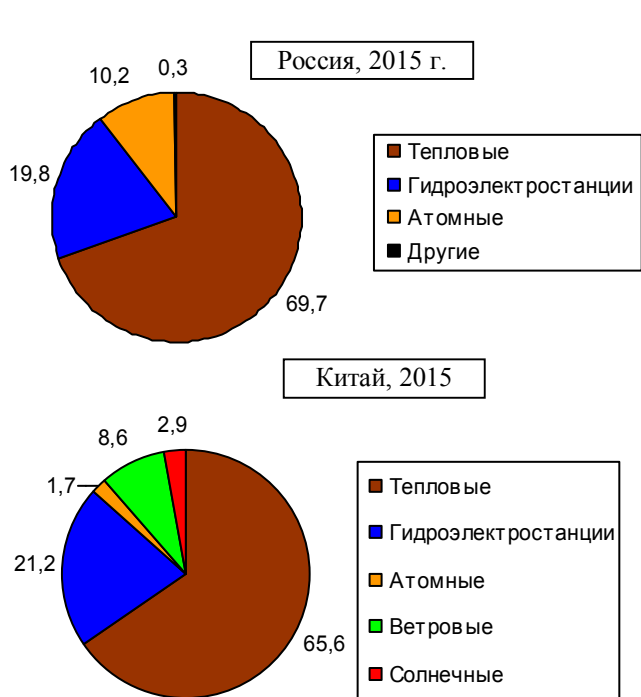
Рис. 1.124, а. Установленная мощность электростанций, млн. кВт. Источники: [1.4, 1.6]; National Bureau of Statistics of China; Japan Statistical Yearbook; U.S. Energy Information Administration (EIA), International Energy; U.S. Census Bureau, Statistical Abstract.
