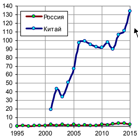
Рис. 1.131. Ввод мощностей по производству электроэнергии, млн. кВт. Источники: [I.6]; National Bureau of Statistics of China.
