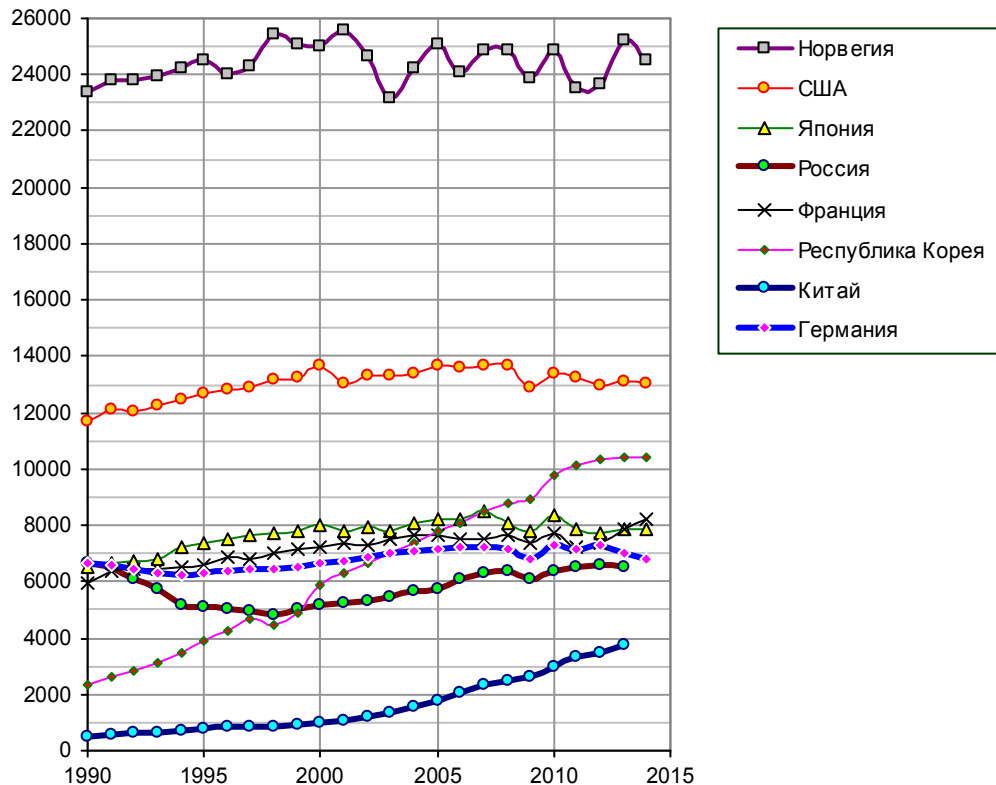
Рис. 1.129. Потребление электроэнергии на душу населения кВт·час/чел. Источник: World Bank, WDI; для 2013 и 2014 гг. – расчет по U.S. Energy Information Administration, EIA.
