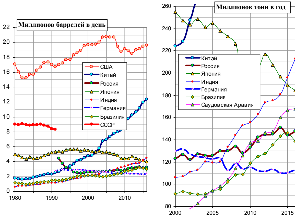
Рис. 1.443. Потребление нефти. Источники: EIA, International Energy Annual; BP Statistical Review of World Energy.
