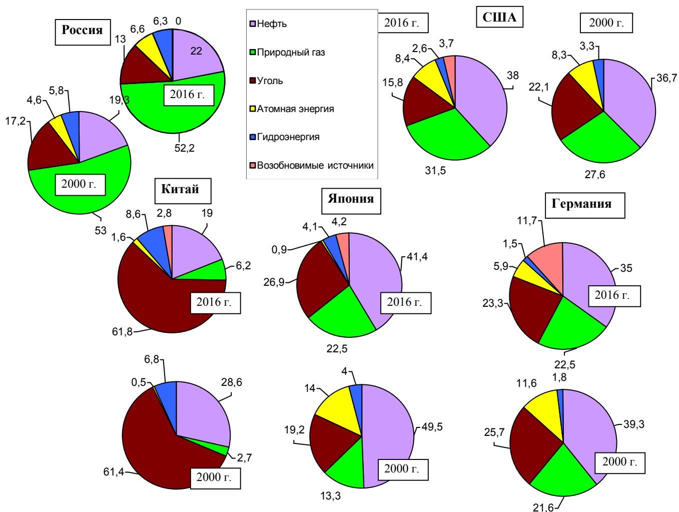
Рис. 1.441. Структура потребления первичной энергии (primary energy) по источникам энергоресурсов (в процентах от общего объема потребления, рассчитанного в Мтое). Источник: по данным BP Statistical Review of World Energy.
