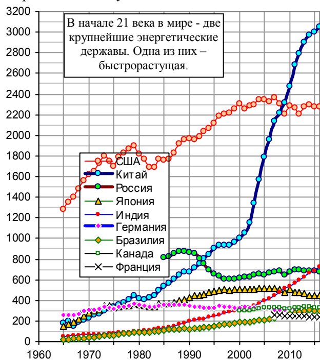
Рис. 1.439, а. Потребление первичной энергии странами – лидерами по этому показателю, млн. тонн условного топлива в нефтяном эквиваленте. Источник: BP Statistical Review of World Energy.
