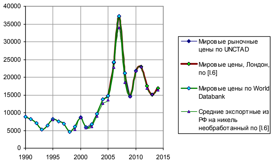
Рис. 1.620. Цены на никель, долл./т. Источники: [1.6]; UNCTAD, Handbook of Statistics; World Bank, World Databank.
