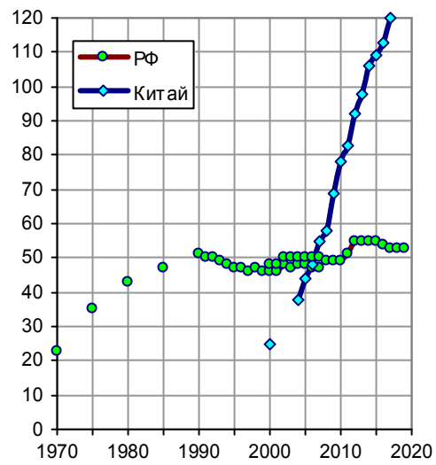
Рис. 1.254. Длина нефтепроводов, тыс. км. Источники: [1.6, 1.7]; BRICS, Joint Statistical Publication.
